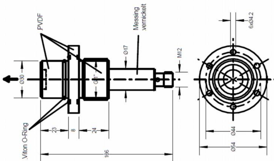
UFA-1500-M30-A-CH / UFA-1500-M30-1P-CH
